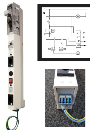
2x T13 16A, 5-pôle
